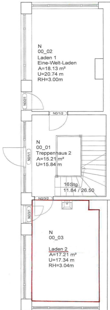
Erdgeschoss
