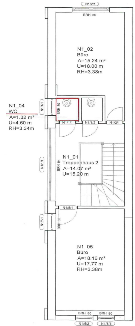
1. Obergeschoss
